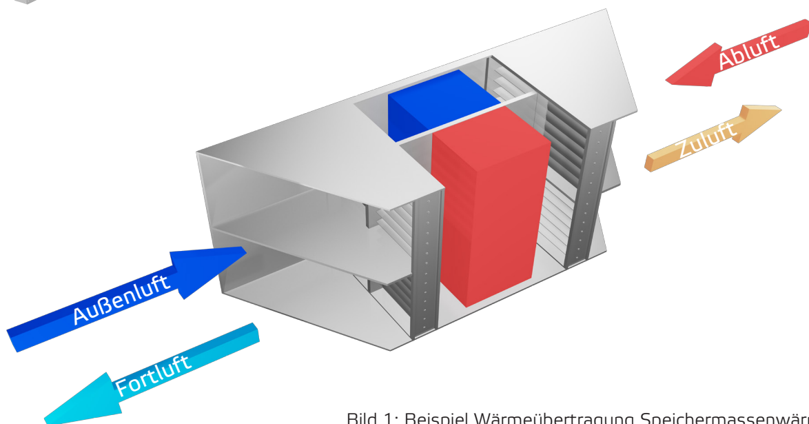
Bild 1: Beispiel Wärmeübertragung Speichermassenwärmetauscher
